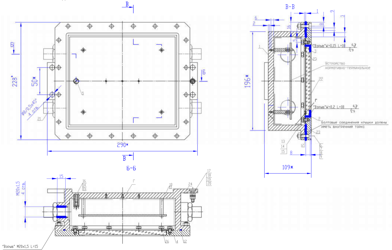
Рис.2. Габаритные и присоединительные размеры.
